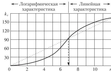
Рис. 3.15. Расходная характеристика клапана MSV-F d = 100 мм
