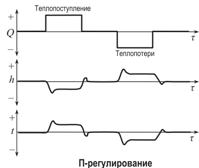
П-регулирование
