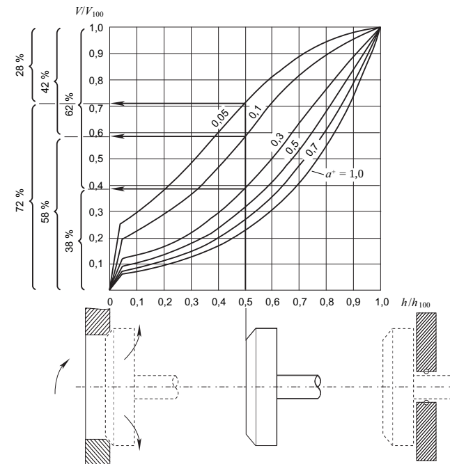
Рис. 4.17. Влияние общего авторитета терморегулятора на потокораспределение
