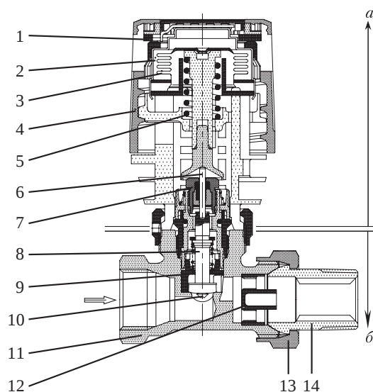
Рис. 4.2. Терморегулятор со встроенным датчиком:
