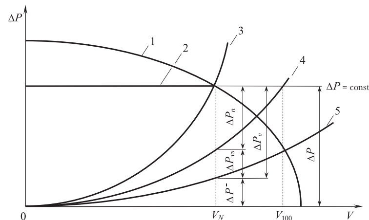
Рис. 3.9. Распределение давлений на регулируемом участке: 1 – характеристика нерегулируемого насоса; 2 – характеристика автоматического регулятора перепада давления; 3 – характеристика регулируемого участка в расчетных условиях; 4 – характеристика регулируемого участка при полностью открытом регулирующем клапане; 5 – характеристика регулируемого участка без учета сопротивления регулирующего клапана
