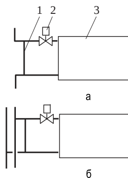
Рис. 4.23. Узлы обвязки теплообменных приборов: а – однокотловых систем; б – двухтрубных систем; 1 – замыкающий участок; 2 – терморегулятор; 3 – теплообменный прибор
