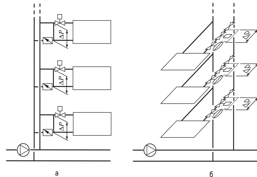
Рис. 3.4. Схемы наилучшего обеспечения работоспособности терморегуляторов
