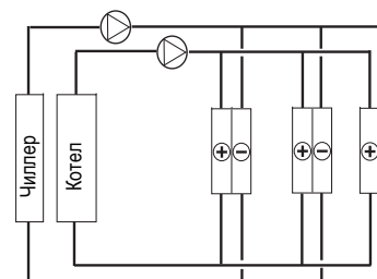
Четырехтрубная система охлаждения и отопления
