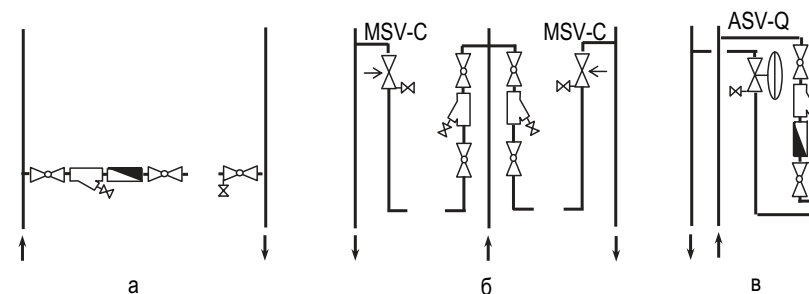
Рис. 9.23. Схемы присоединения однетрубных приборных веток
