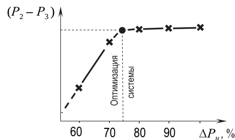
Рис. 11.7. Определение рабочей точки насоса
