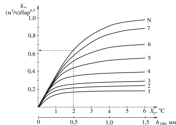
Рис. 4.21. Влияние настройки дросселя на пропускную способность терморегулятора
