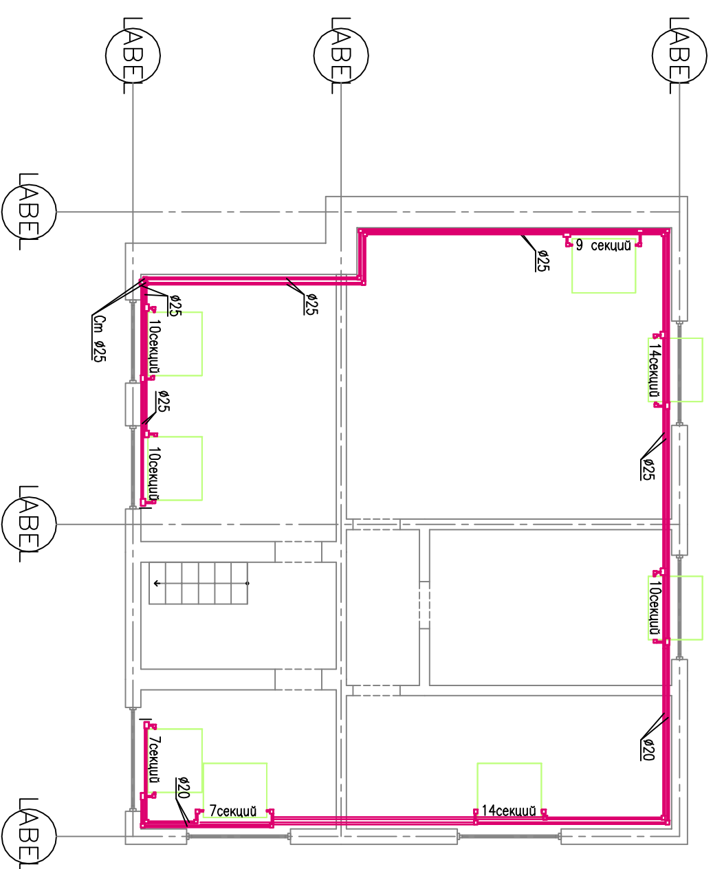
Второй этаж
