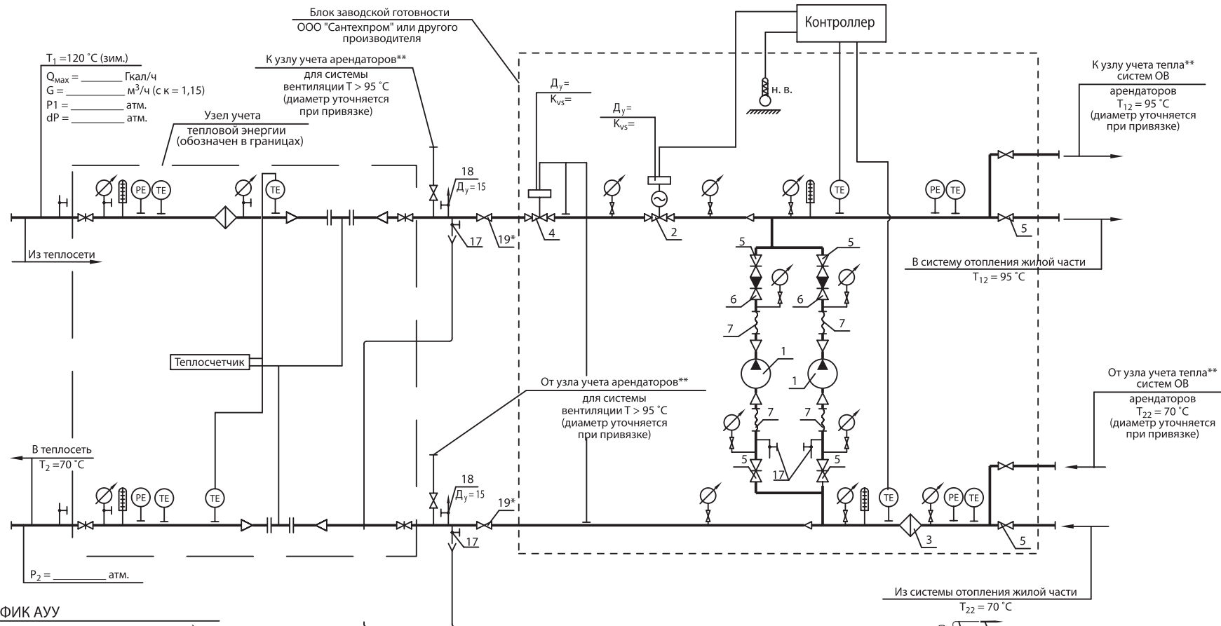
Схема № 8. ПРИНЦИПИАЛЬНАЯ СХЕМА АВТОМАТИЗИРОВАННОГО УЗЛА УПРАВЛЕНИЯ С НАСОСАМИ СМЕШЕНИЯ НА ПЕРЕМЫЧКЕ ДЛЯ ТЕМПЕРАТУРЫ ДО АУУ t = 120\text{—}70\text{ }^{\circ}\text{C} , ПРИ ОДНО- И ДВУХТРУБНЫХ СИСТЕМАХ ОТОПЛЕНИЯ С ТЕРМОСТАТАМИ ( P1 - P2 \geq 12\text{ м вод. ст.} )
