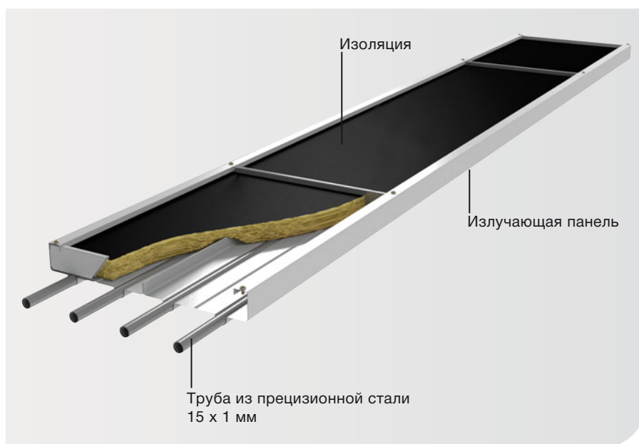
Рис. 1. Отдельный модуль ZIP
