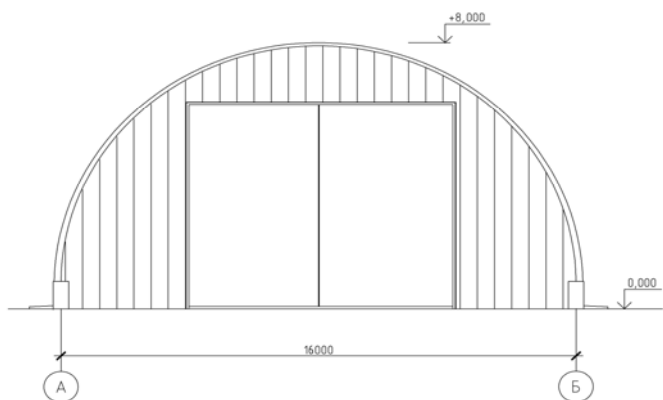
Фасад А-Б
