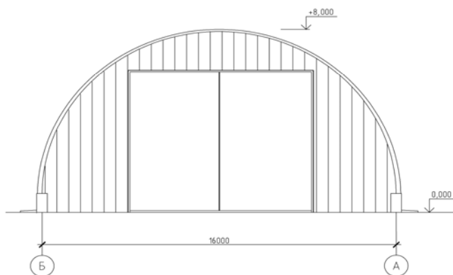
Фасад Б-А
