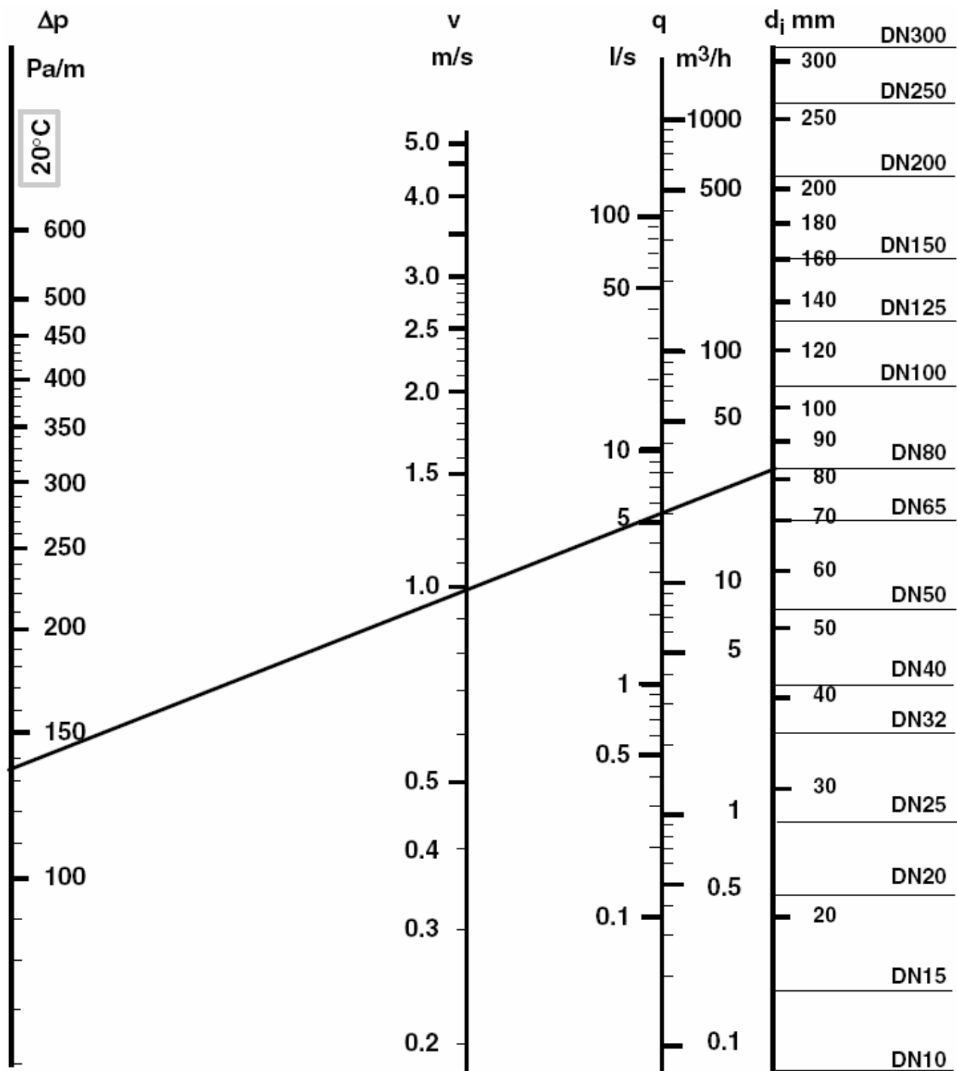
Рисунок С1 Падение давления и скорость воды при температуре 20^\circ\text{C} (в стальной трубе с коэффициентом шероховатости 0.05\text{ mm} ).
