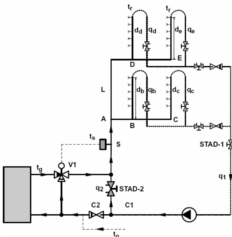
Рисунок 7.8а Насос рециркуляции поддерживает температуру воды
