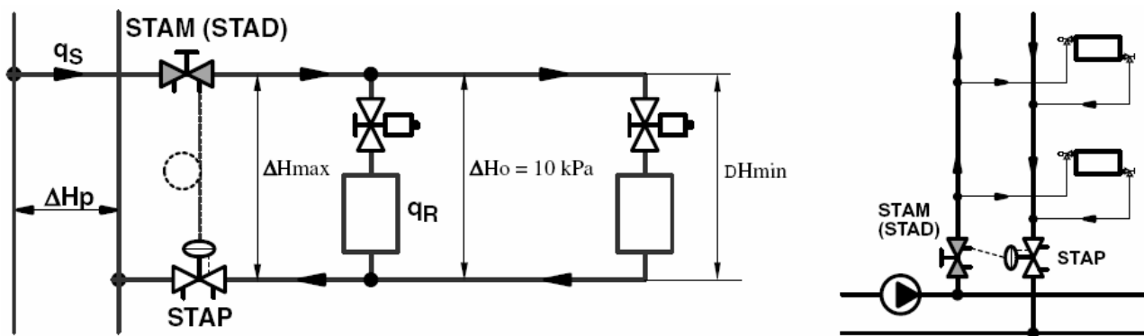
Рисунок F10. STAP удерживает перепад давления на входе контура постоянным.
