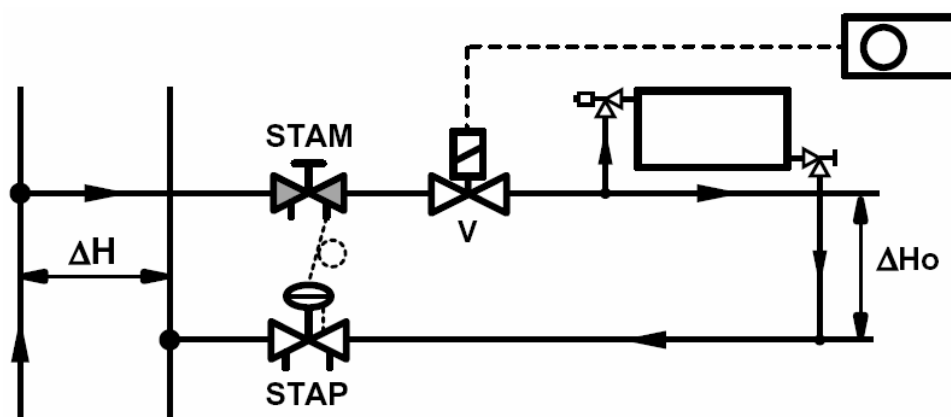
Рисунок 7.4b Неверный проект с расположением управляющего клапана после измерительного клапана STAM
