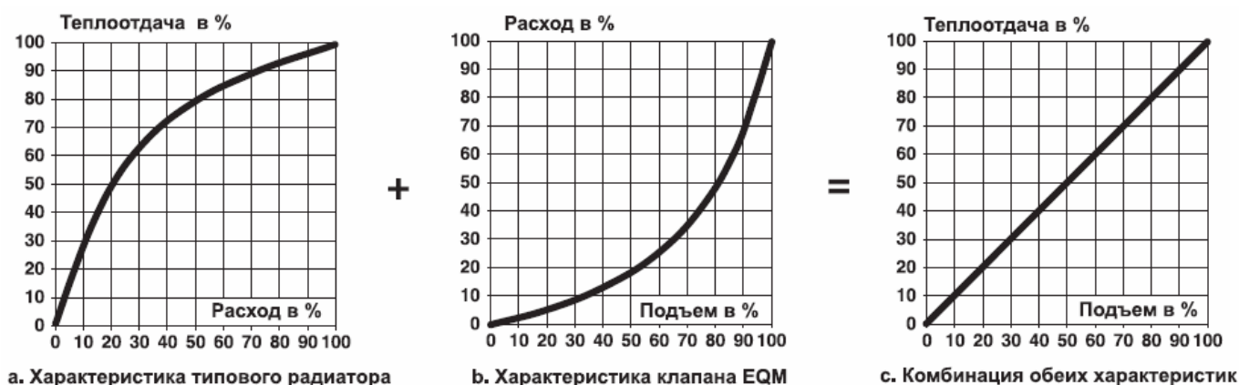
Рисунок F4. Нелинейность характеристики радиатора компенсируется установкой регулирующего клапана с инверсной нелинейной характеристикой.
