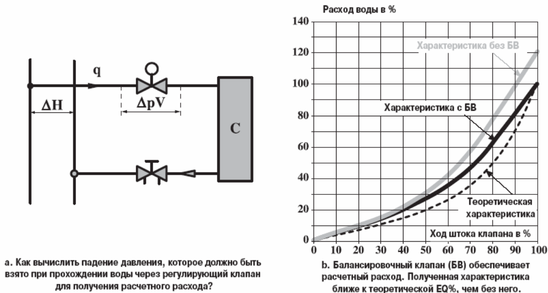
Рисунок F6. Если размер регулирующего клапана завышен, балансировочный клапан улучшает характеристику регулирующего клапана.
