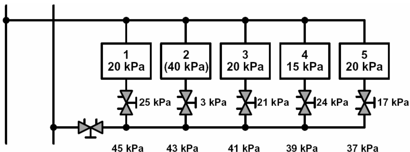
Рисунок 5.7 Перепад давления по все контурам и потери давления на балансирующих клапанах и терминалах.
