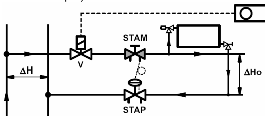
Рисунок 7.4с Управляющий клапан расположен перед измерительным клапаном STAM
