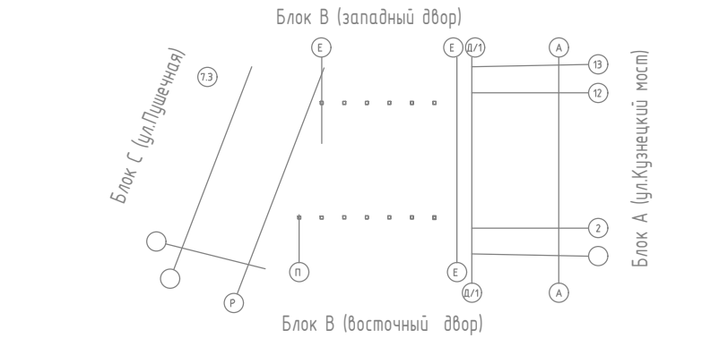
Фрагмент плана промежуточного этажа ЛК5
