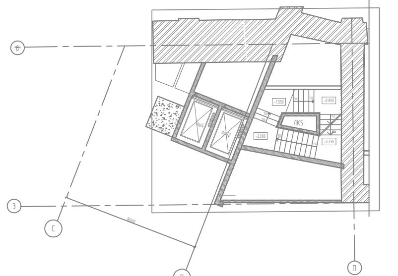
Фрагмент плана промежуточного этажа ЛК5
