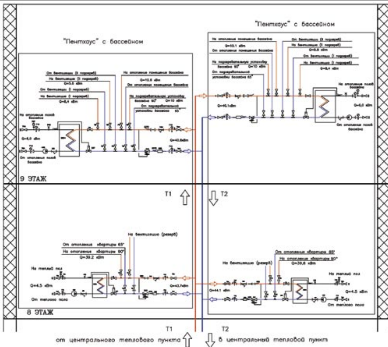
рис. 2. Проектное решение оснащения «пентхаусов» 8-9 этажей
