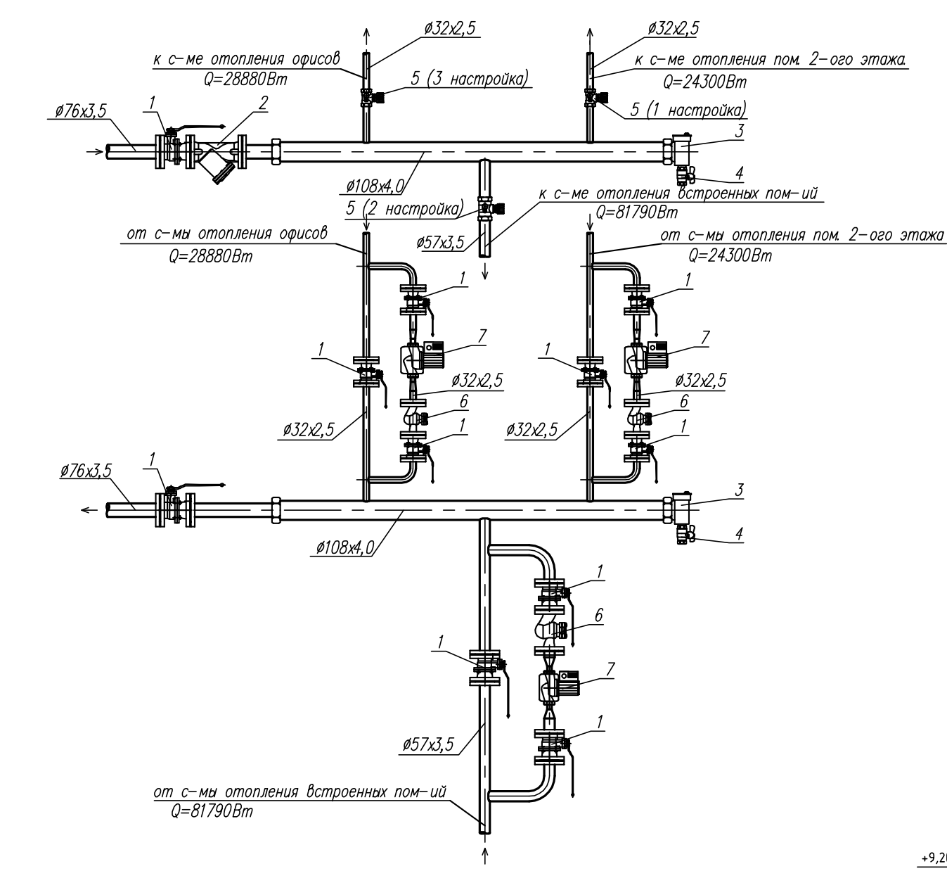
Схема распределительного коллектора
