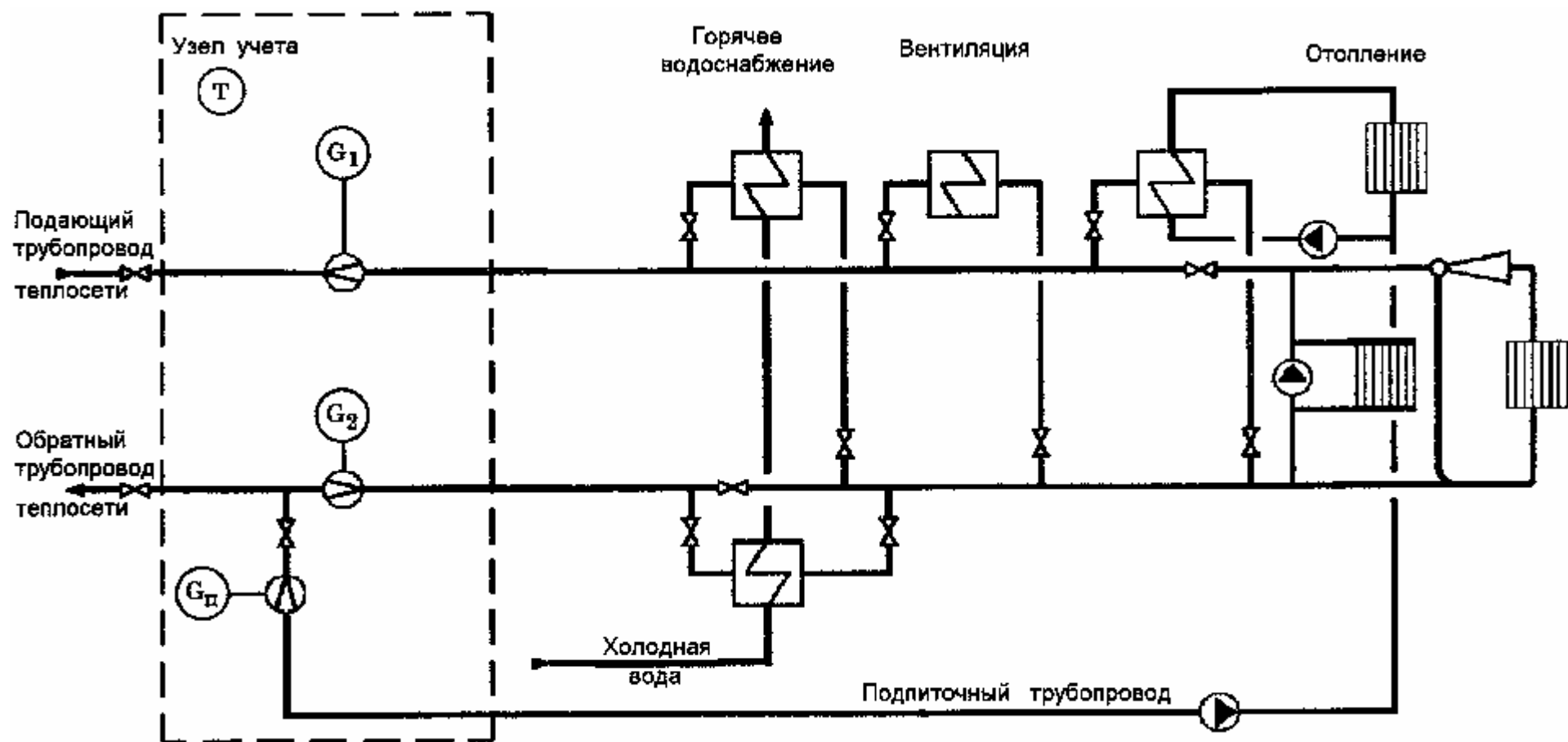
Рис. 8. Принципиальная схема размещения точек измерения количества тепловой энергии и массы (объема) теплоносителя, в закрытых системах теплоснабжения с суммарной тепловой нагрузкой, не превышающей 0,1 Гкал/ч.
