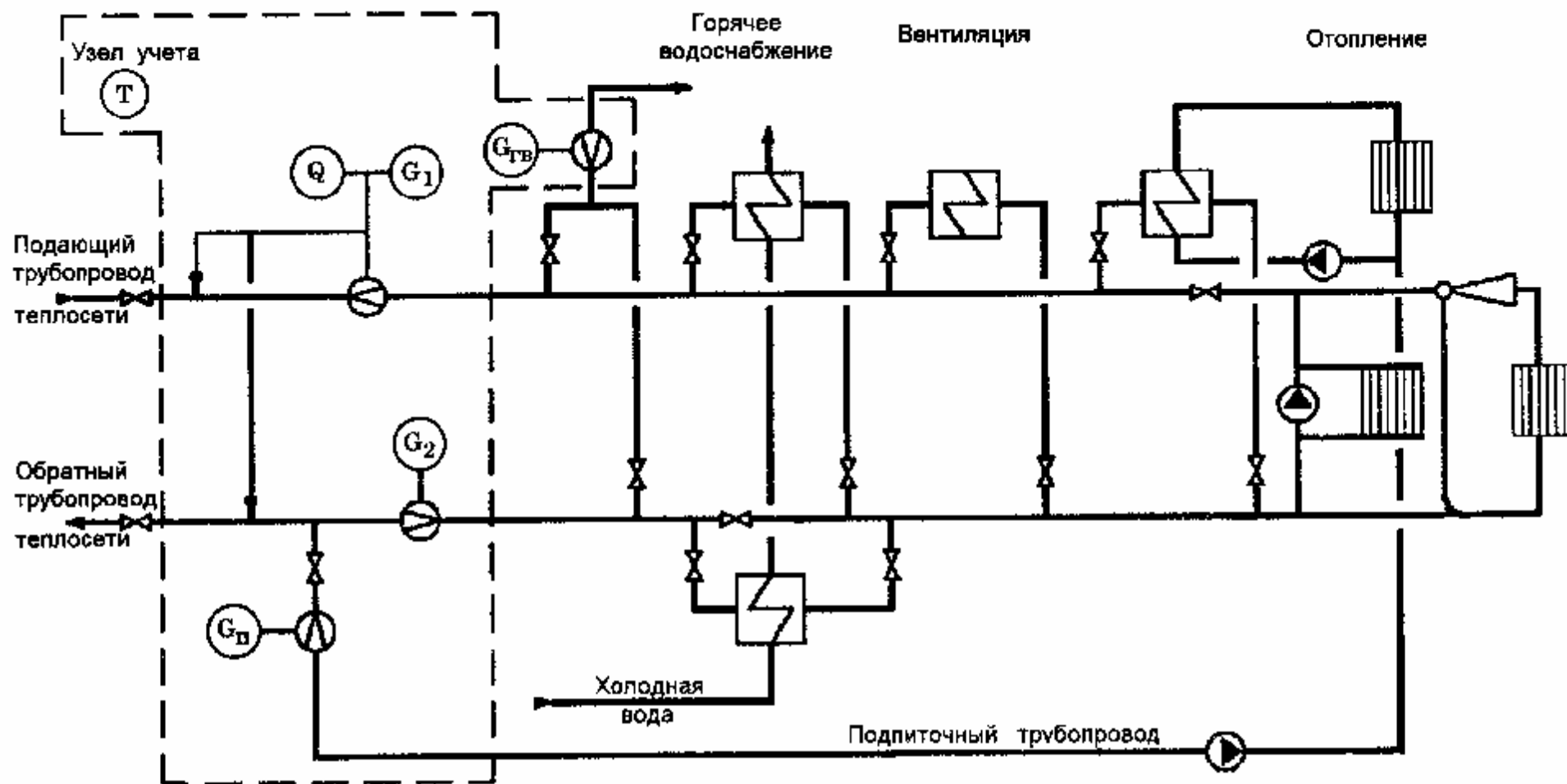
Рис. 5. Принципиальная схема размещения точек измерения количества тепловой энергии и массы (объема) теплоносителя, в открытых системах теплоснабжения с суммарной тепловой нагрузкой, не превышающей 0,5 Гкал/ч.
