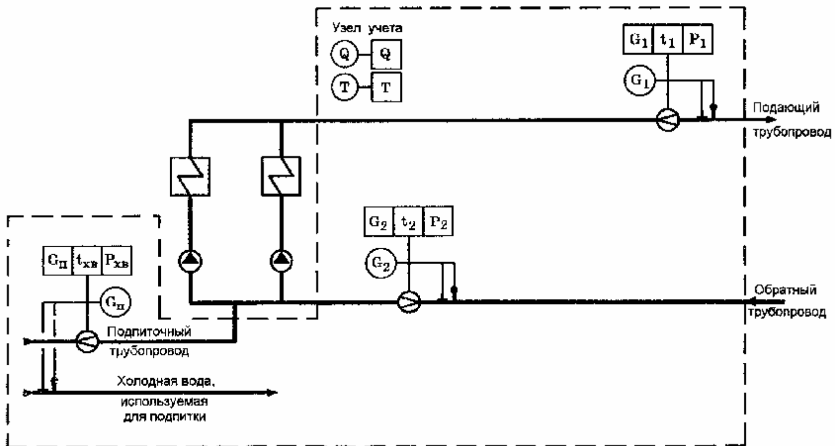
Рис. 1. Принципиальная схема размещения точек измерения массы (объема) теплоносителя и его регистрируемых параметров на источнике теплоты для водяных систем теплоснабжения.
