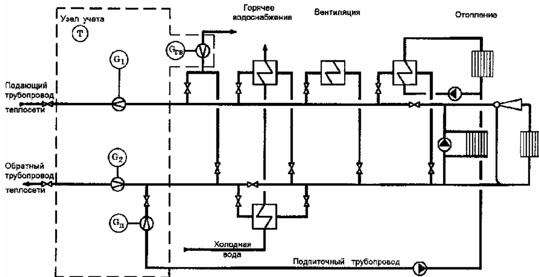
Рис. 7. Принципиальная схема размещения точек измерения количества тепловой энергии и массы (объема) теплоносителя, в открытых системах теплоснабжения с суммарной тепловой нагрузкой, не превышающей 0,1 Гакл/ч.
