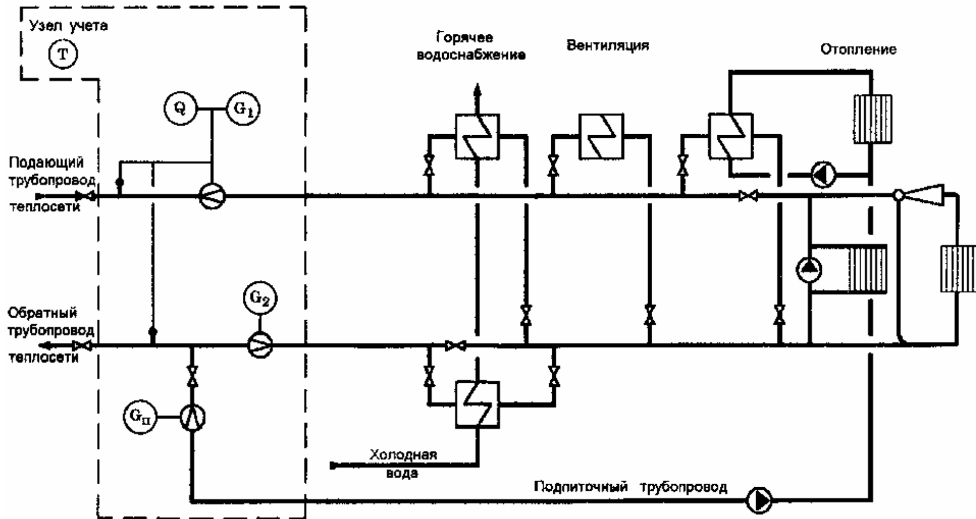
Рис. 6. Принципиальная схема размещения точек измерения количества тепловой энергии и массы (объема) теплоносителя, в закрытых системах теплоснабжения с суммарной тепловой нагрузкой, не превышающей 0,5 Гкал/ч.
