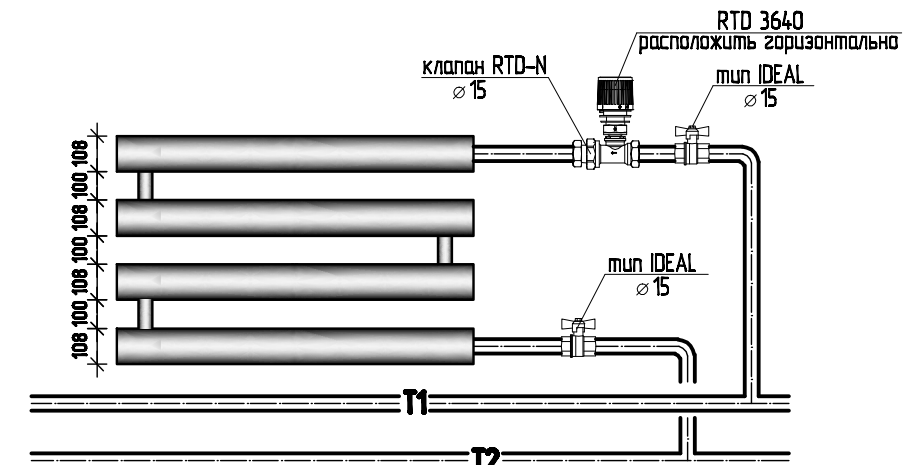
Узел обвязки отопительных приборов.
