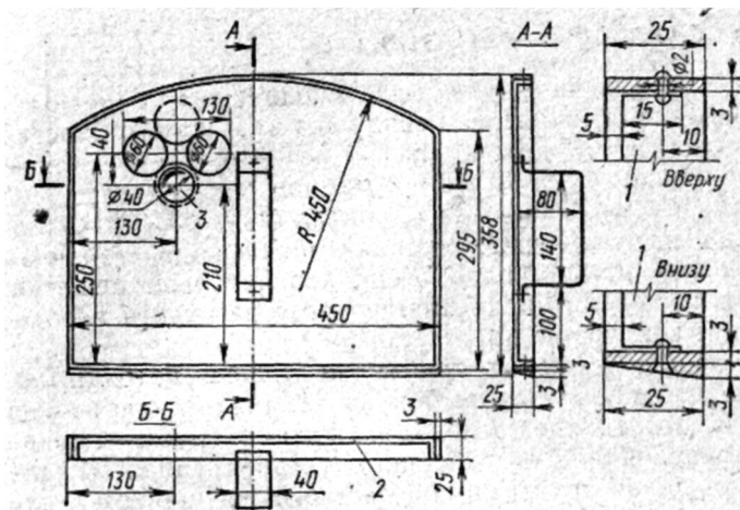
Рис. 11. Заслонка печей «Теплушка-2» и «Теплушка-4»:
