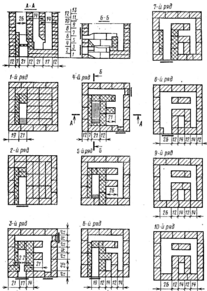
Рис 49. Кладки рядов 1...10 печи «Двухъярусный колпак» размером 102X102 см для угля. Остальные ряды выкладывают из красного кирпича по чертежу печи для дров. (Размеры в см)
