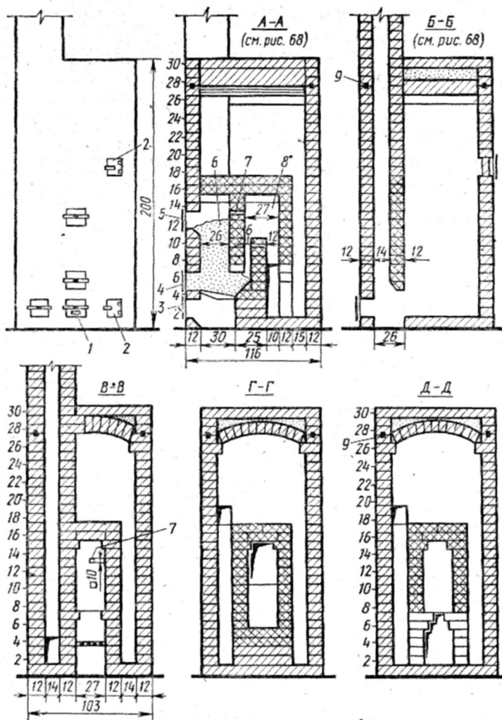
Рис. 68. Разрезы печи длительного горения:
