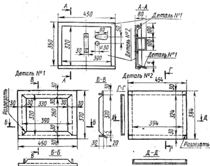
Рис. 26. Заслонка печи "Теплушка-10" из кровельного железа толщиной 1 мм. Разрезы б-б, в-в, г-г и д-д условно показаны для деталей с отогнутыми краями. Пунктир — линии сгиба. (Размеры в мм)
