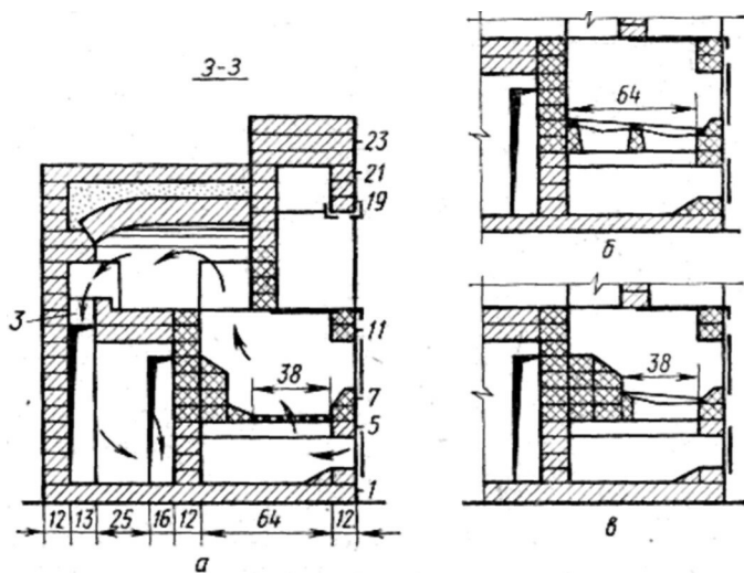
Рис. 36. Кладка топливника печи «Теплушка-15» размером 154X141 см для разных видов топлива: а - дров и торфа; б - для подмосковного угля; в - для антрацита и каменного угля. (Размеры в см)
