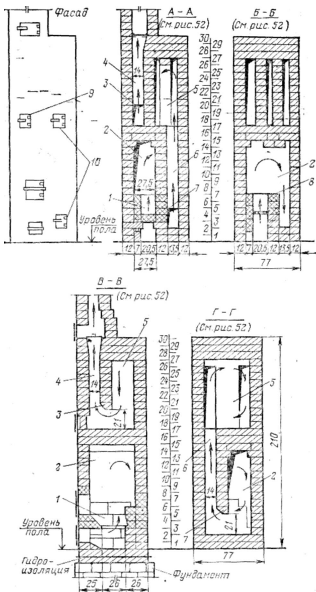
Рис. 51. Разрезы отопительной печи "Двухъярусный колпак" размером 77x77 см. Позиции расшифрованы на рисунках 47, 48. (Размеры в см)
