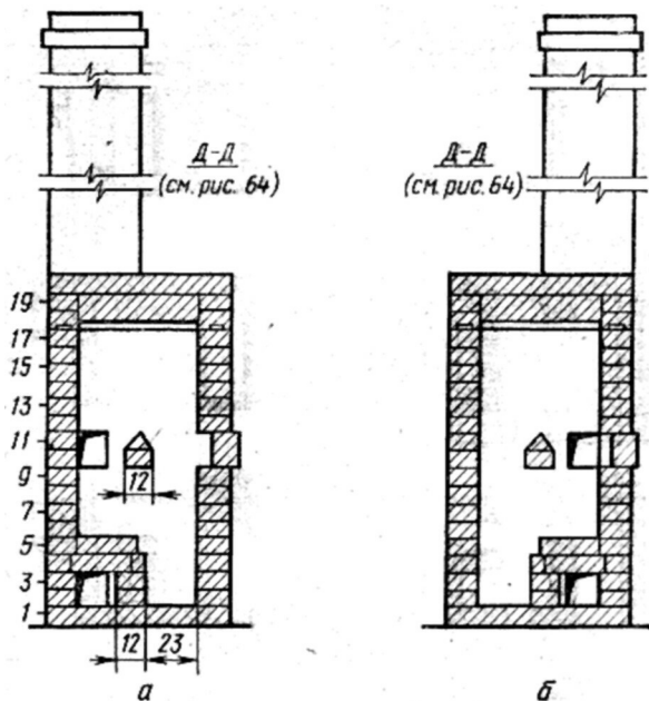
Рис. 65. Разрезы кухонного очага «Колпаковый» при левом основном (а) и правом (б) расположении трубы
