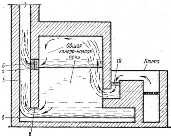
Рис. 16. Схема движения дымовых газов для обогрева камеры печи по выходе из-под плиты в «Теплушке-4»: а — уровень пода; б — уровень второго ряда; в — подvertка трубы
