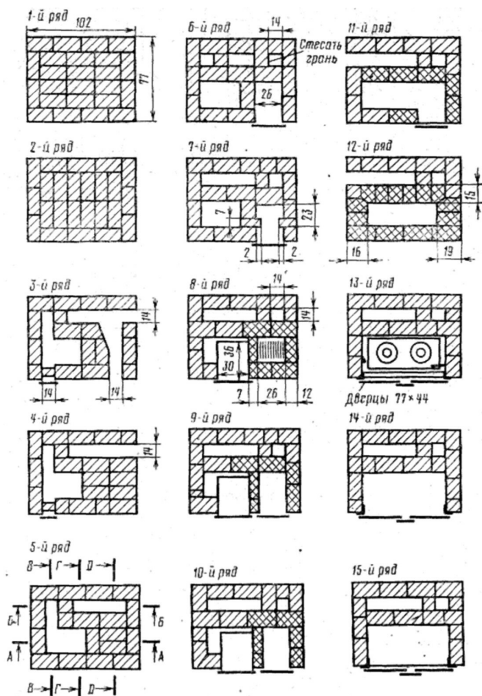
Рис. 60. Кладки 1...31 рядов печи "ИП-2". Разрезы показаны на рисунке 59. (Размеры в см)
