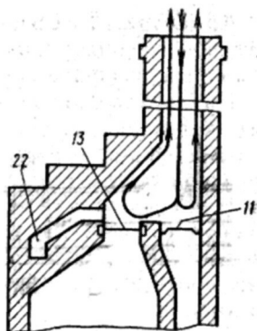
Рис. 9. Схема движения воздуха в дымовой трубе выше закрытой вьюшки
