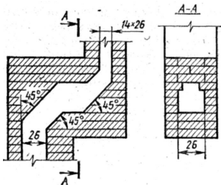
Рис. 7. Образец устройства бора. (Размеры в см)
