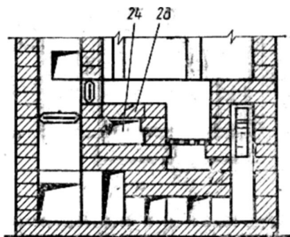
Рис. 21. Разделение топок печи «Теплушка-9» и ее плиты.
