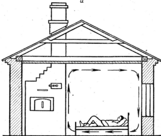
Рис. 5. Схемы движения воздуха в помещении, отапливаемом обычной русской печью ( a ) и «Теплушкой» ( б )
