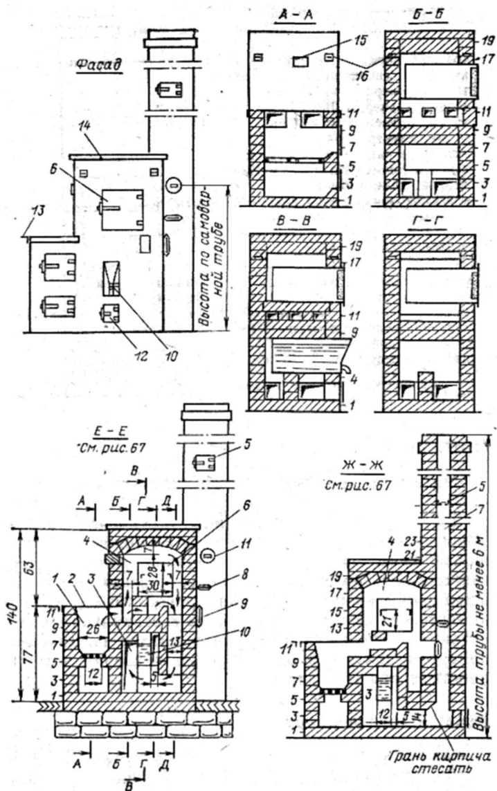
Рис. 64. Разрезы кухонного очага «Колпаковый»:
