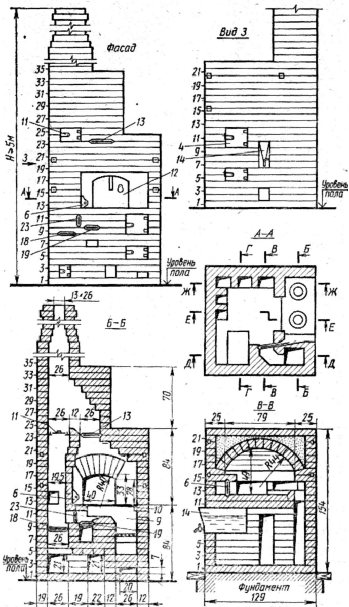
Рис. 19. Разрезы русской печи «Теплушка-4» размером 129X129 см. (Размеры в см)
