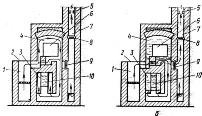
Рис. 62. Схемы движения в кухонном очаге «Колпаковый» горячих дымовых газов (а) и холодного воздуха в прогретом очаге (б); пунктирная линия—просачивание холодного воздуха через щели закрытой задвижки:
