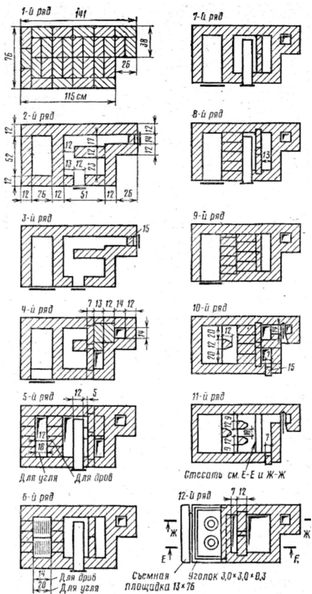
Рис 67. Кладки 1...21 рядов кухонного очага «Колпаковый». (Размеры в см)
