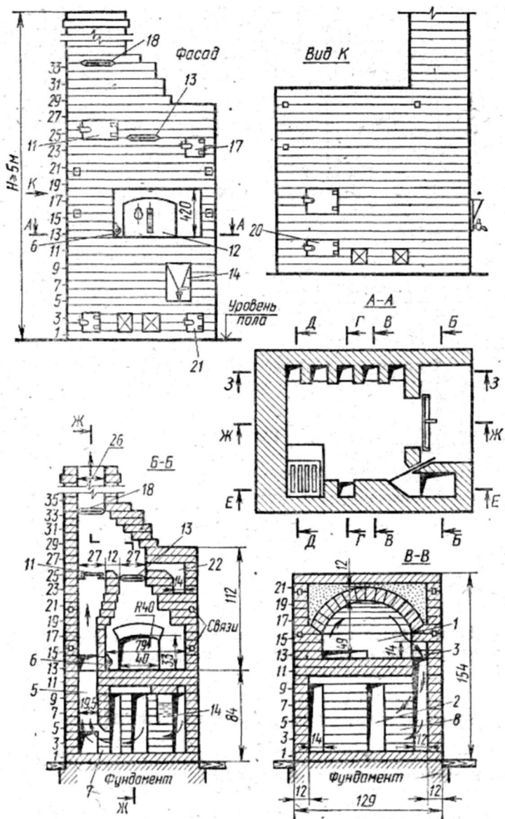
Рис. 12. Разрезы русской печи «Теплушка-2»
