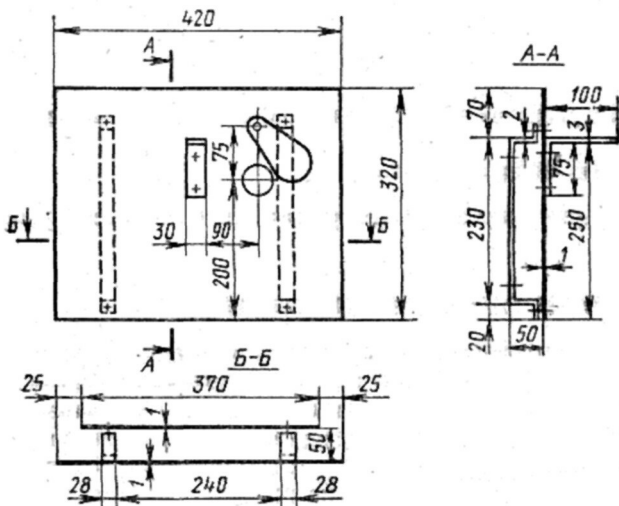
Рис. 34. Заслонка для печи «Теплушка-15» размером 154X141 см. (Размеры в мм)
