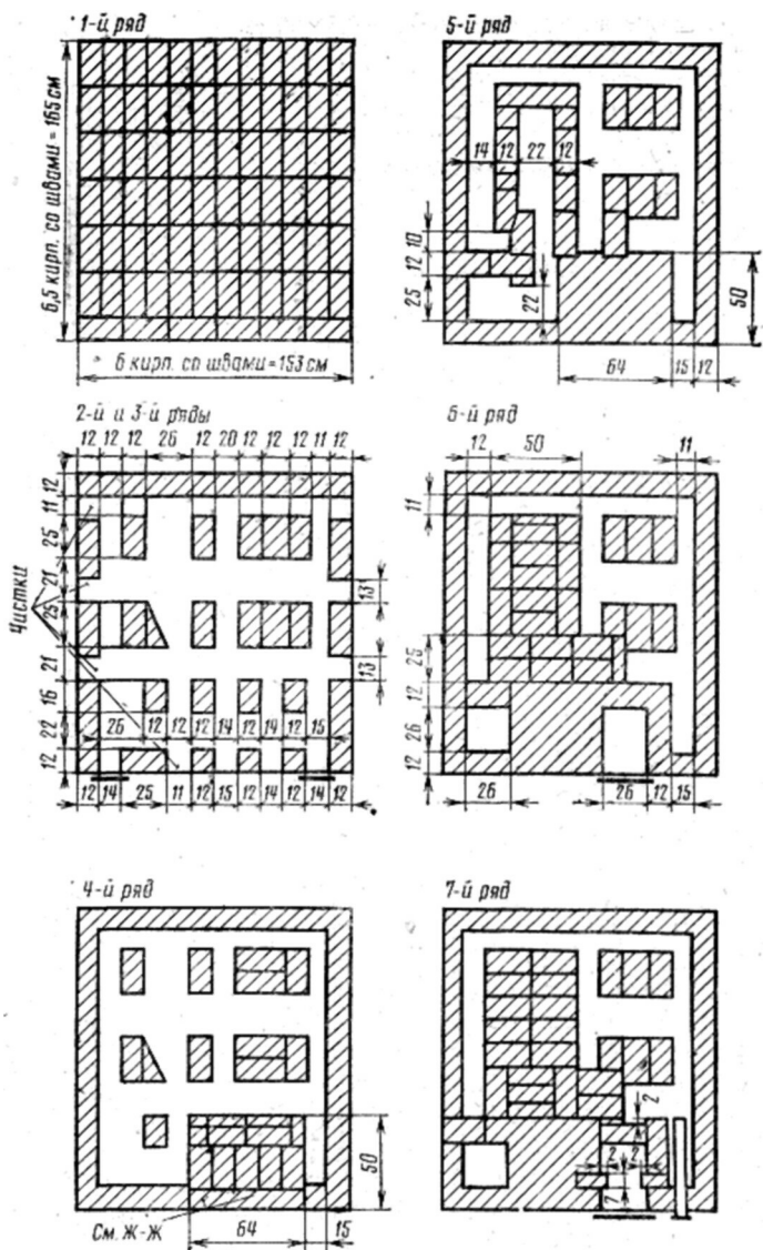
Рис. 23. Кладки 1...28 рядов печи «Теплушка-9». (Размеры в см)
