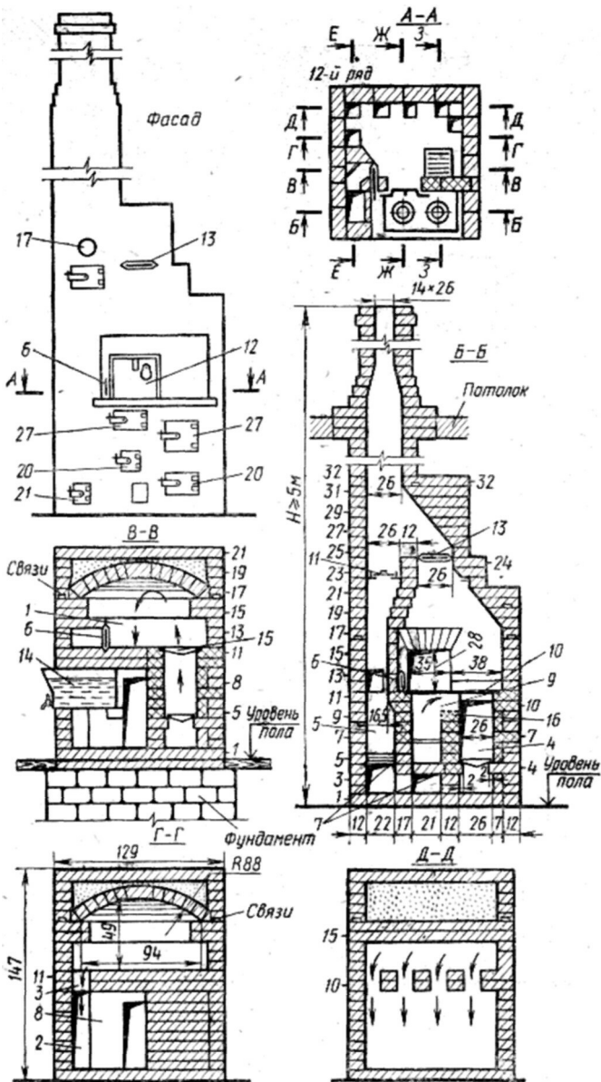
Рис. 30. Разрезы русской печи «Теплушка-15» размером 129×129 см. (Размеры в см)
