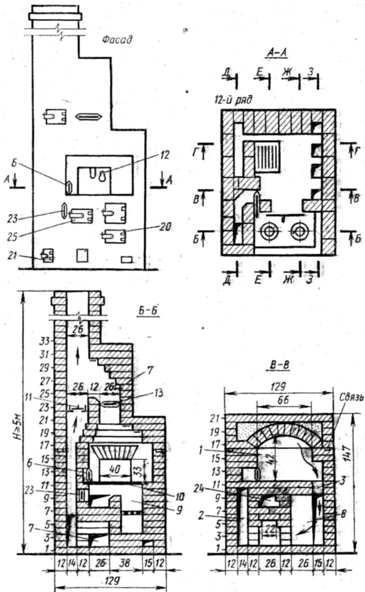
Рис. 27. Разрезы русской печи "Теплушка-10". (Размеры в см)
