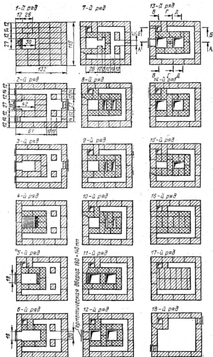
Рис. 69. Кладки 1...31 рядов печи длительного горения. Разрезы показаны на рисунке 67. (Размеры в см)
