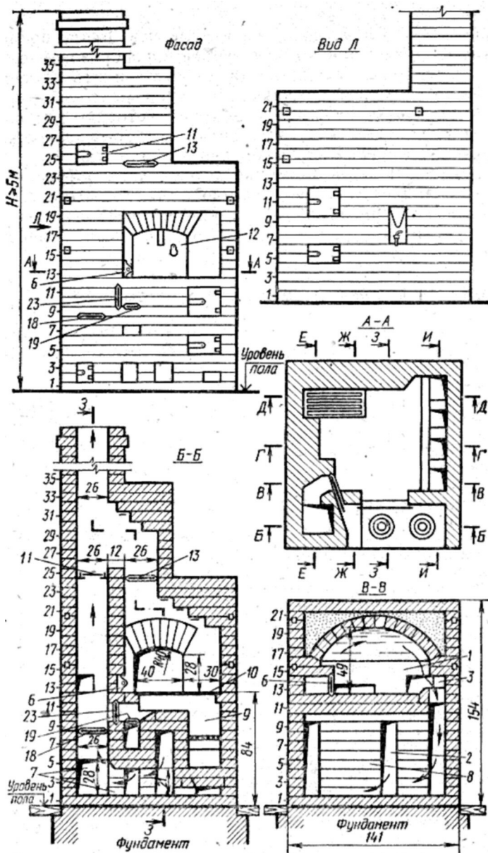
Рис. 17. Размеры русской печи «Теплушка-4» размером 154X X141 см. (Размеры в см)
