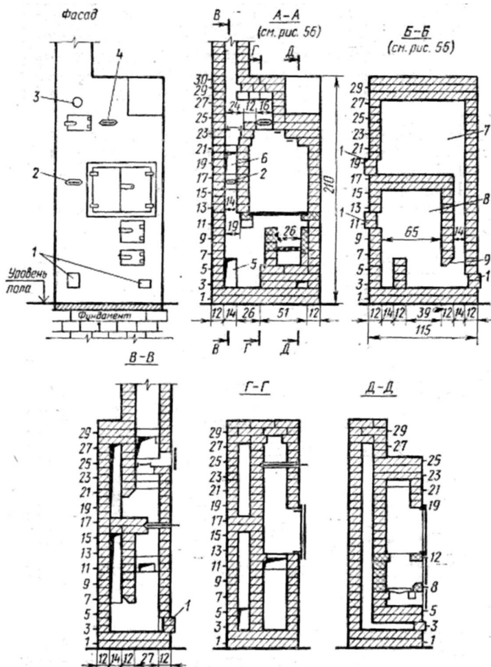
Рис. 55. Разрезы отопительно-варочной печи «ИП-1»:
