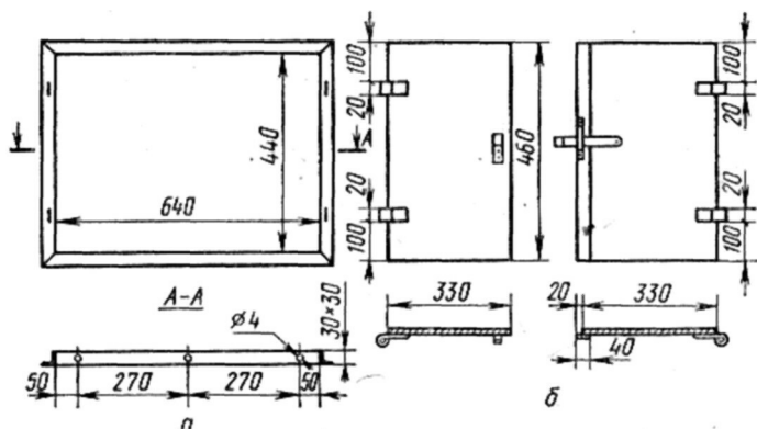
Рис. 54. Дверца отопительно-варочной печи «ИП-1»:
