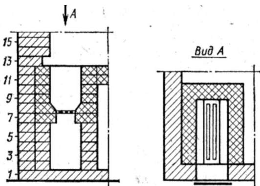
Рис. 6. Тип топливника для горизонтальной укладки дров
