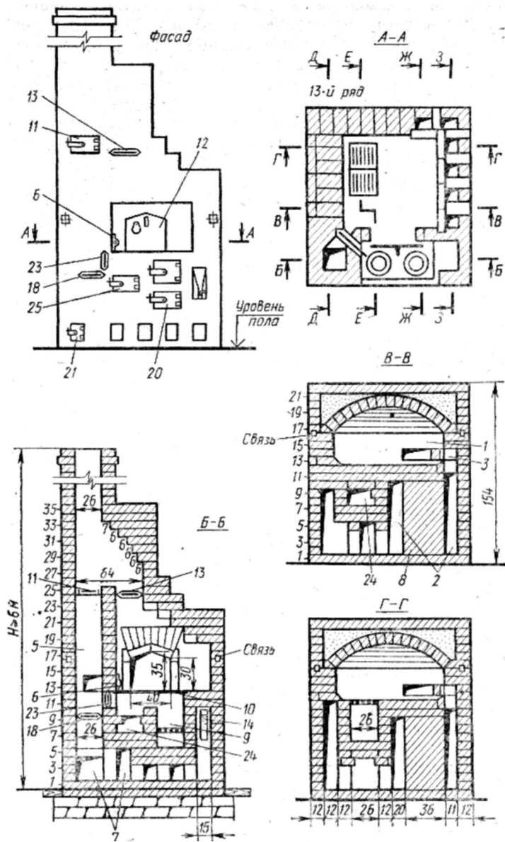
Рис. 23. Разрезы русской печи «Теплушка-9». (Размеры в см)
