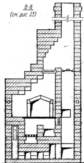
Рис. 24. Разрез русской печи «Теплушка-9» с трубой справа
