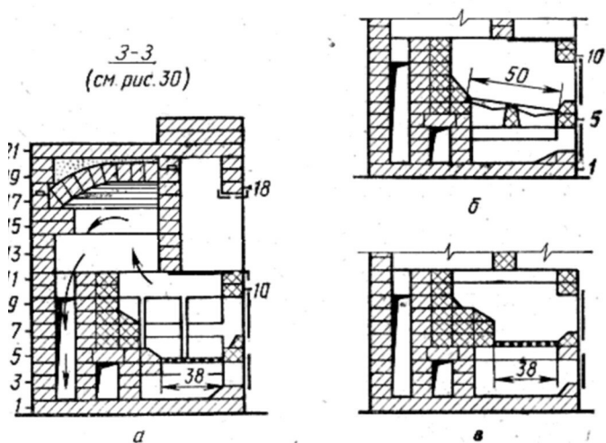
Рис. 31. Кладка топливника печи «Теплушка-15» размером 129X129 см для разных видов топлива:
