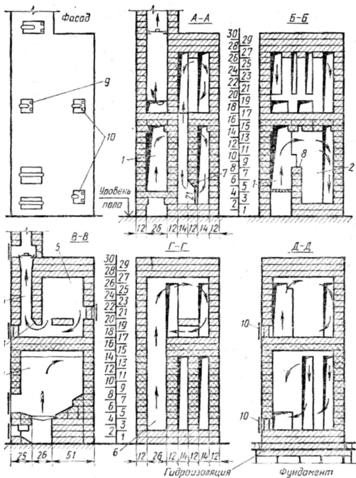
Рис. 48. Разрезы отопительной печи «Двухъярусный колпак» размером 102×102 см:
