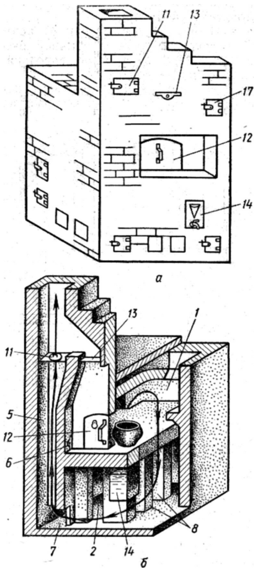
Рис. 3. Общий (а) и внутренний (б) виды русской печи "Теплушка-2"
