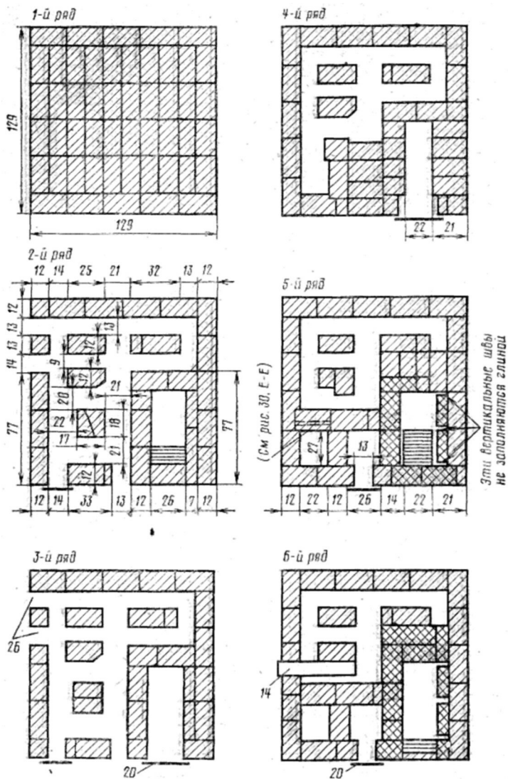
Рис 33. Кладки 1...33 рядов печи «Теплушка-15» размером 129x129 см. Кладка с шестого ряда топливника ведется по вертикальному разрезу для соответствующего вида топлива. (Размеры в см)
