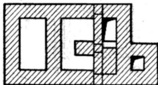
Рис. 66. Варианты кладок рядов при правом расположении трубы:
