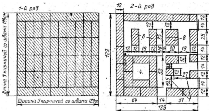
Рис. 14. Кладки 1 и 2-рядов печи «Теплушка-2» размером 129×129 см. (Размеры в см)
