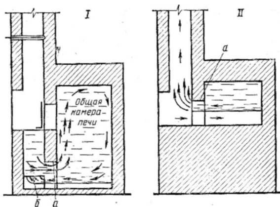
Рис. 42. Схемы движения дымовых газов для обогрева общей камеры печи «Теплушка-5» (I) и при топке обычной русской печи (II):
