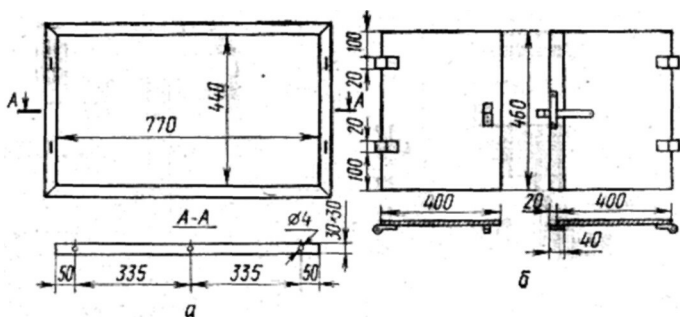
Рис. 58. Дверца отопительно-варочной печи «ИП-2»:
