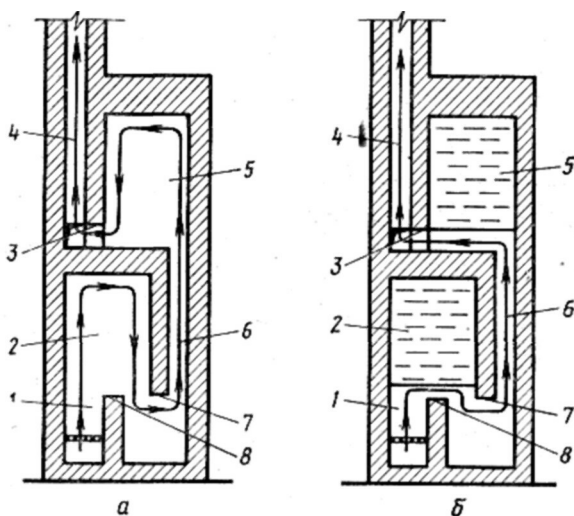
Рис. 47. Основная принципиальная схема устройства печи «Двухъярусный колпак». Стрелками указано направление движения горячих газов (а) и холодного воздуха в прогретой печи (б):
