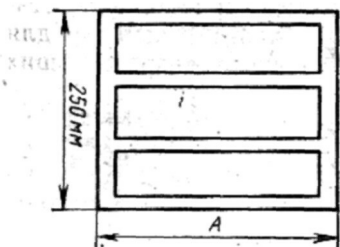
Рис. 8. Съемная облегченная колосниковая решетка. (Размер «А» различен для разных «Теплушек»)
