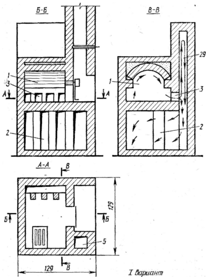
Рис. 16. Разрезы русской печи «Теплушка-7»
