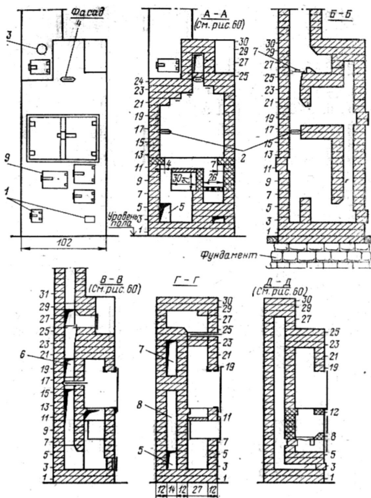
Рис. 59. Разрезы отопительно-варочной печи «ИП-2»: 1.. 8 — см. на рисунке 65; 9 — духовой шкаф. (Размеры в см)
