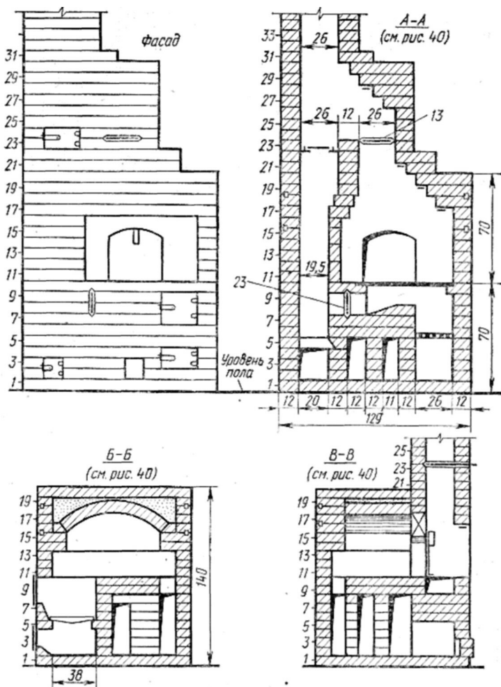
Рис. 39. Разрезы русском печи «Теплушка-3». (Размеры в см)
