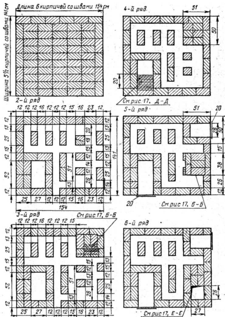
Рис. 18. Кладки 1...35 рядов печи «Теплушка-4» размером 151X141 см. (Размеры в см)
