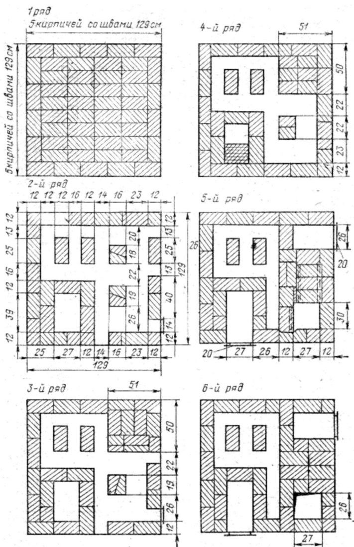
Рис. 20. Кладки 1...35 рядов печи «Теплушка-4» размером 129 × 129 см. (Размеры в см)
