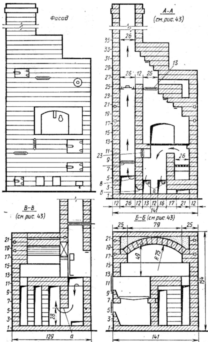
Рис. 41. Разрезы русской печи «Теплушка-3»: а, б, в — подвертки. (Размеры в см)
