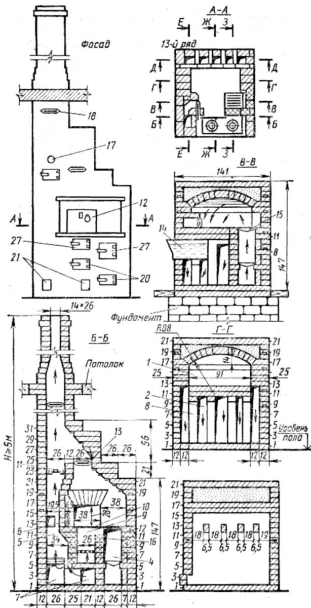
Рис. 35. Разрезы русской печи «Сплушка-15» размером 154x141 см. (Размеры в см)
