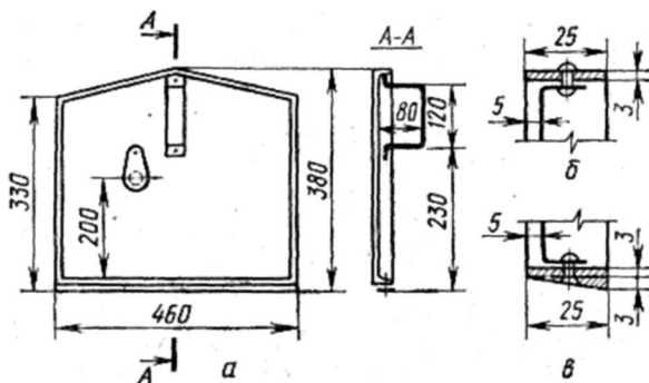
Рис. 22. Заслонка печи «Теплушка-9» (а), крепление листа к раме вверху (б) и внизу (в). (Размеры в мм)
