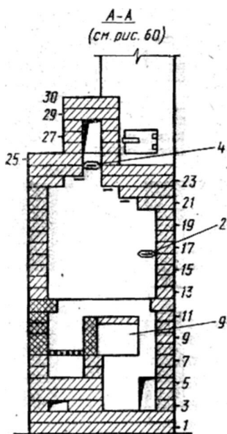
Рис. 61. Разрез А—А печи "ИП-2" с трубой справа, кладка третьего ряда. Позиции расшифрованы на рисунках 55 и 59. (Размеры в см)
