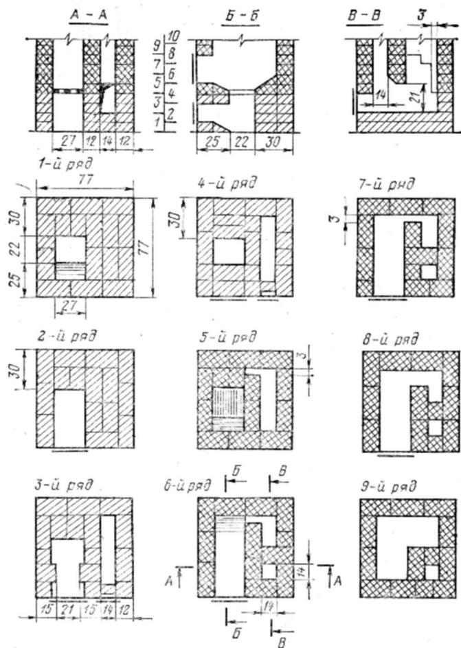
Рис. 52. Кладки 1...9 рядов печи «Двухъярусный колпак» размером 77×77 см для дров. Остальные ряды выкладывают по чертежу печи для угля: по 14-й ряд включительно из огнеупорного кирпича, а выше — из красного кирпича. (Размеры в см)
