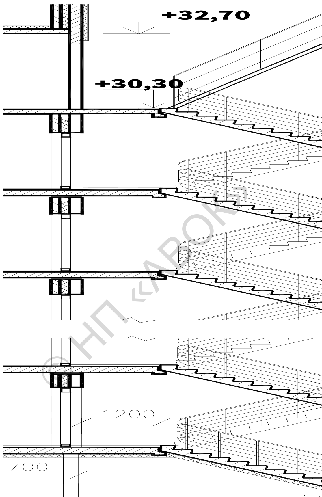
Рис. П-3. Разрез по лестничной клетке жилого дома
