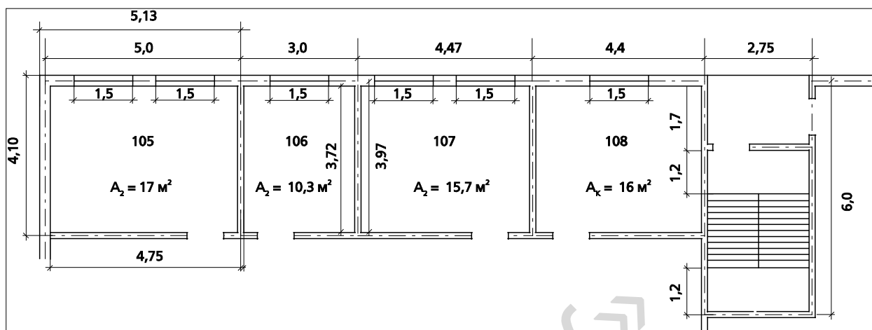
Рис. П-2. Фрагмент плана типового этажа жилого дома
