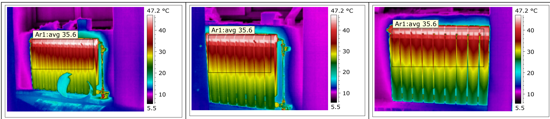
Радиаторы в помещении бассейна под соот. окнами (слева направо).
