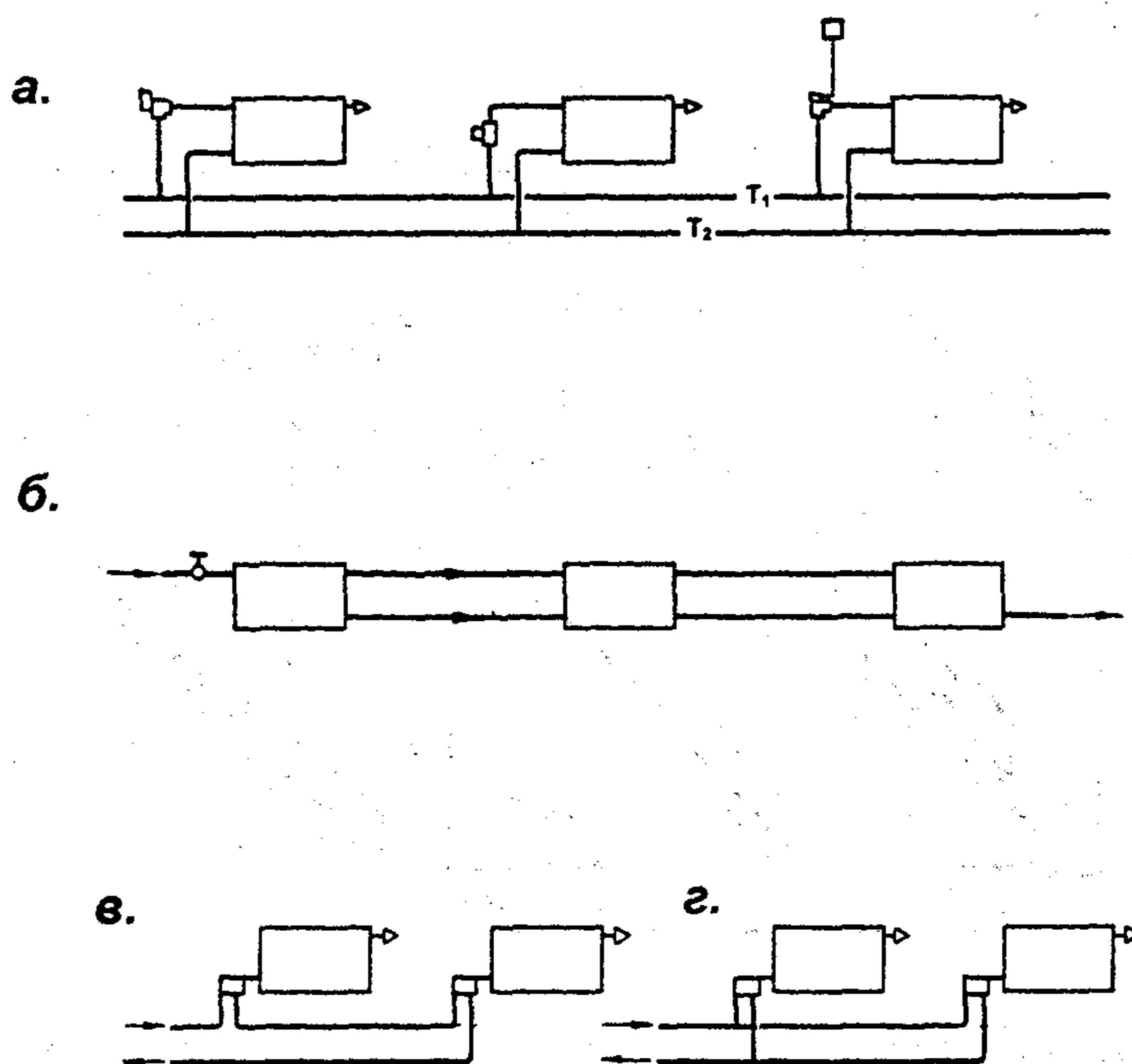
Рис. 2.3. Схемы ветвей горизонтальных систем водяного отопления: а – двухтрубная с термостатами; б – однотрубная проточная; в, г, – однотрубная и двухтрубная с четырёхходовыми узлами нижнего подключения
