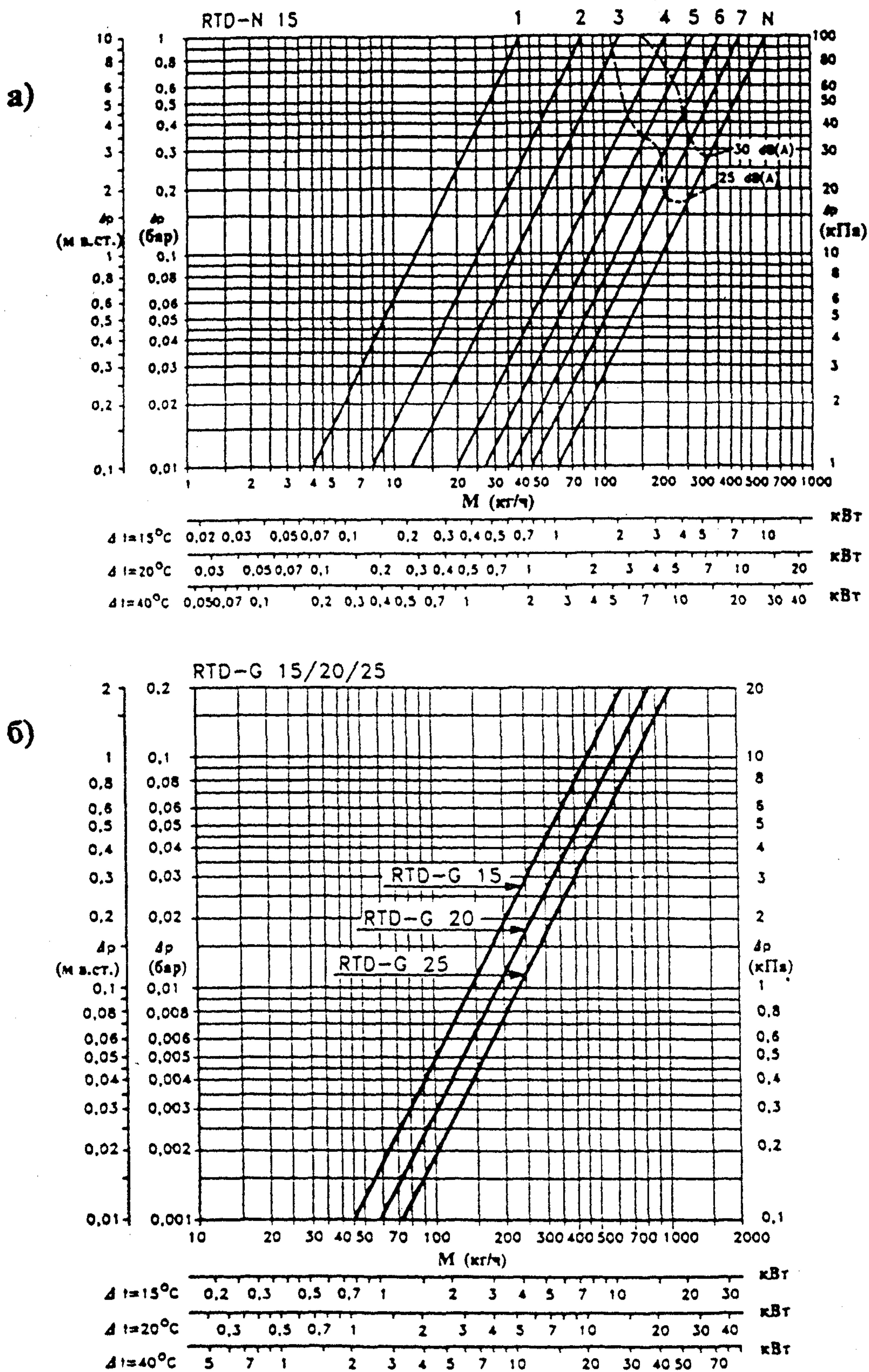
Рис. 2.6. Гидравлические характеристики термостатов «Данфосс»: а) RTD-N 15 при различных уровнях настройки клапана для двухтрубных систем отопления с подводками d_y 15 мм; б) RTD-G для гравитационных и насосных однетрубных систем отопления с подводками d_y 15, 20 и 25 мм
