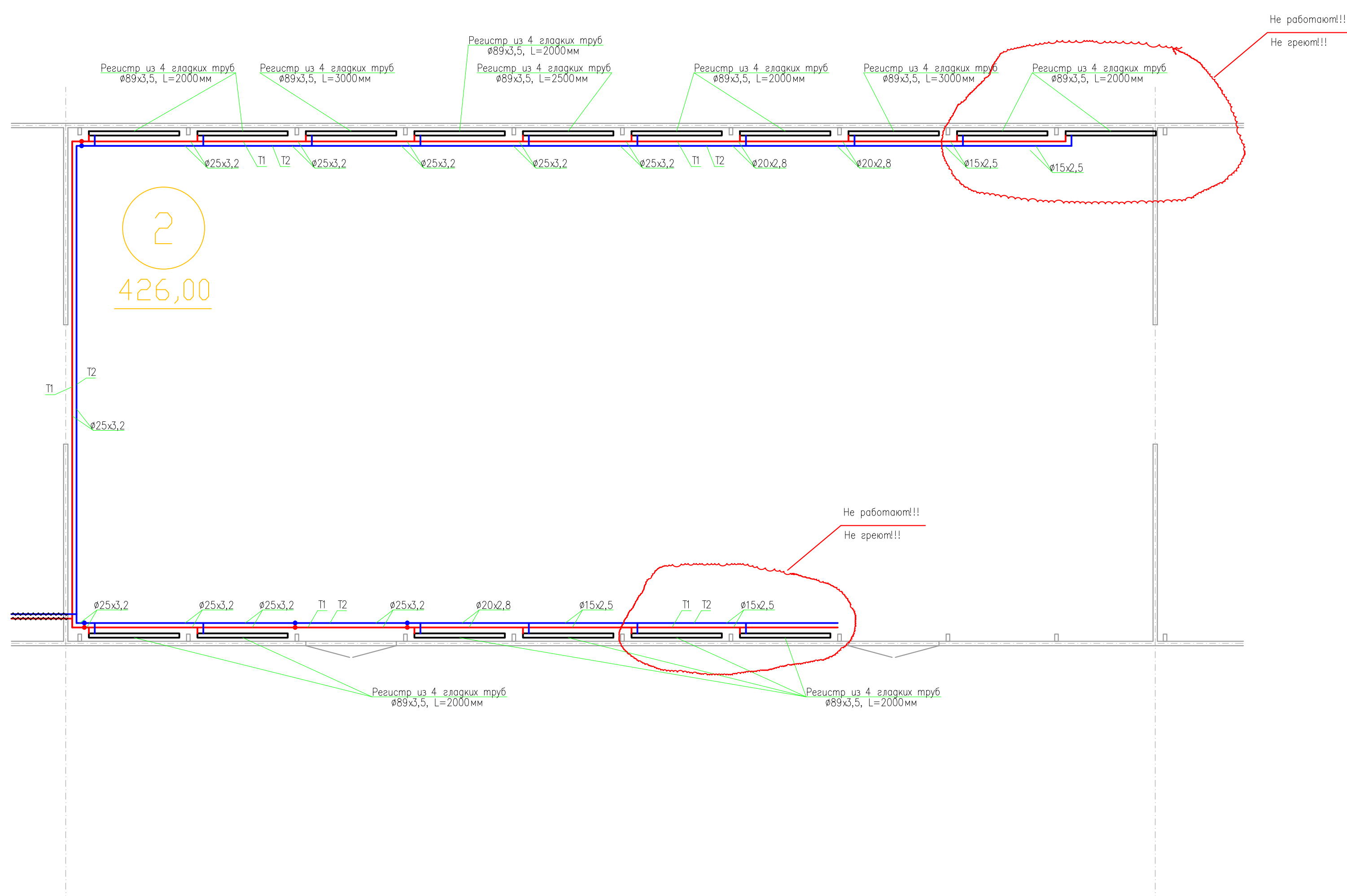
План системы радиаторного отопления
